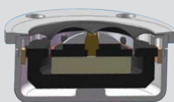
Oben: Die einzigartig konstruierte Membran des EWB Hochtöners endet in der Mitte auf einem Metallstift
